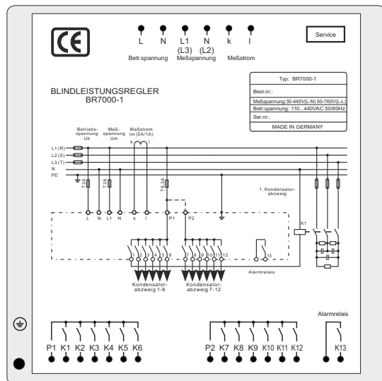
Bild 2: BR 7000-1 Rückansicht
