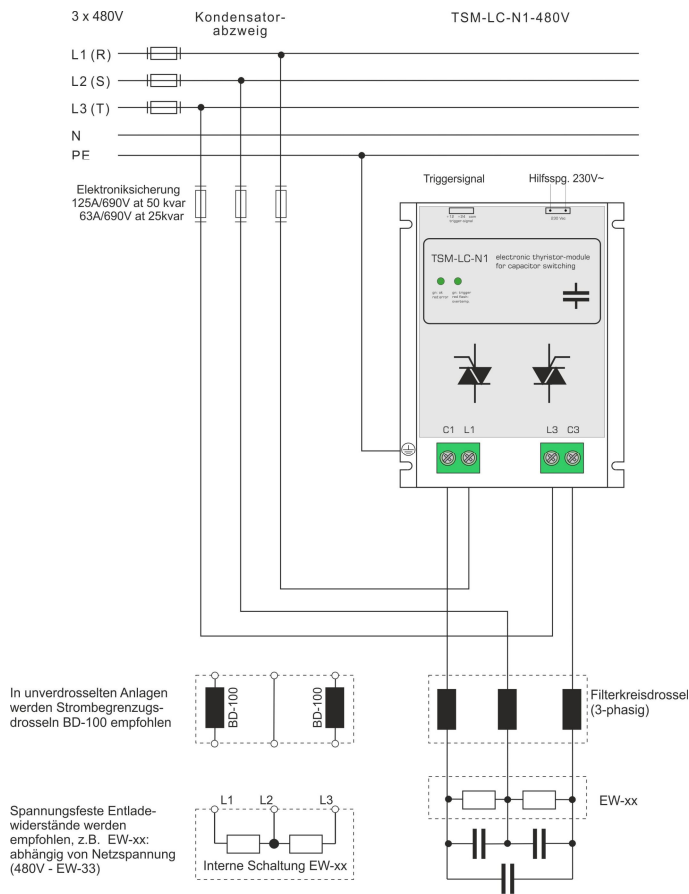
Bild 1: Anschlußplan dreiphasige Last (Standard)
